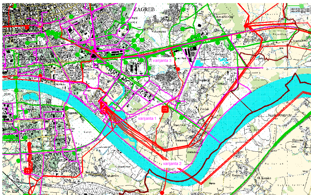
Slika 4.2.2. Trasa cjevovoda od TE-TO do budućeg CGO, prikaz varijantinih rješenja na izvadku iz Nacrta prijedloga ID PP GZ, kartografski prikaz 2. Infrastrukturni sustavi i mreže, 2.A. Energetski sustav, umanjeni prikaz
